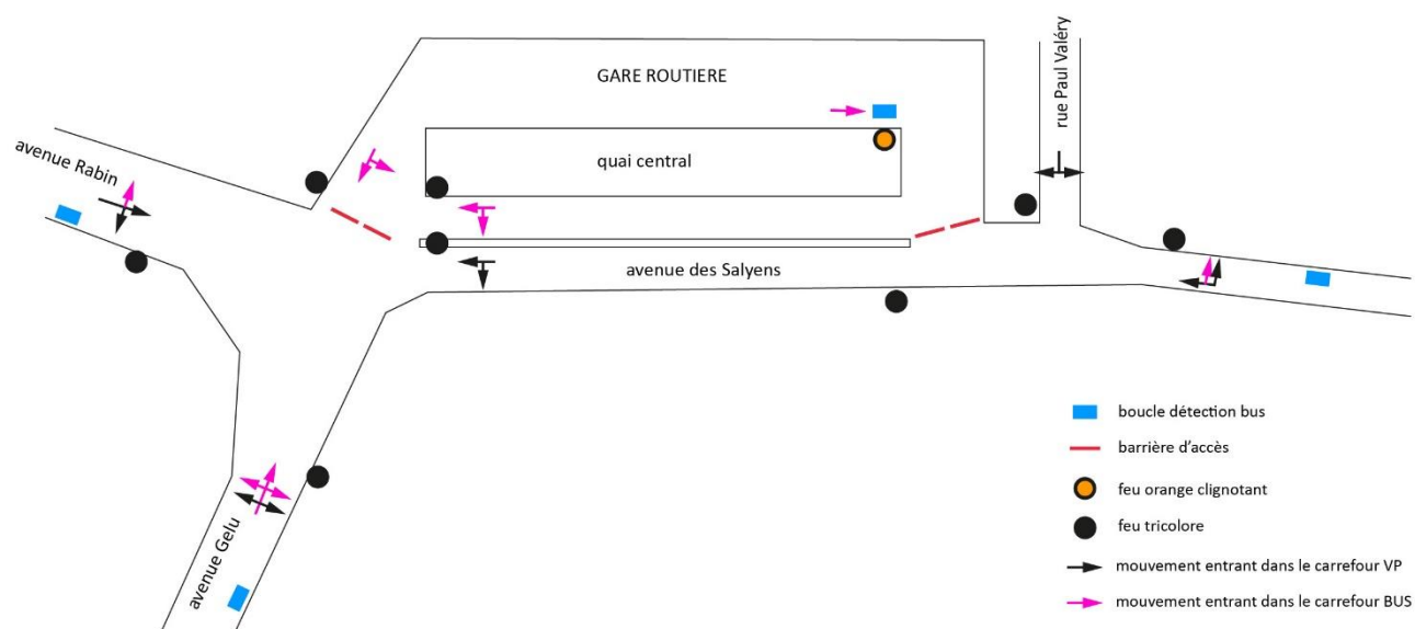
Plan schématique d'implantation des feux
