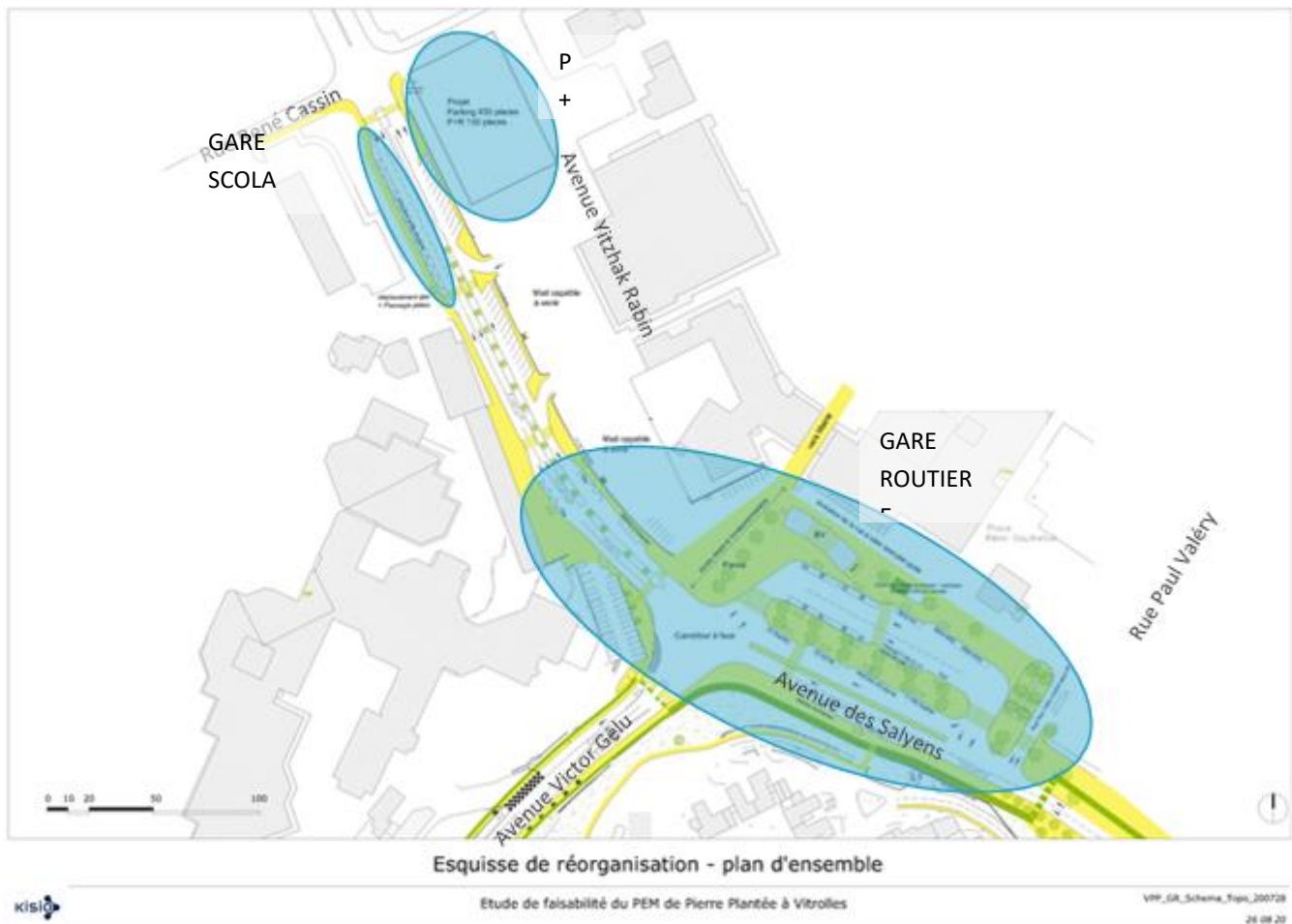
Plan de situation de la gare routière, de la gare scolaire et du P+R
