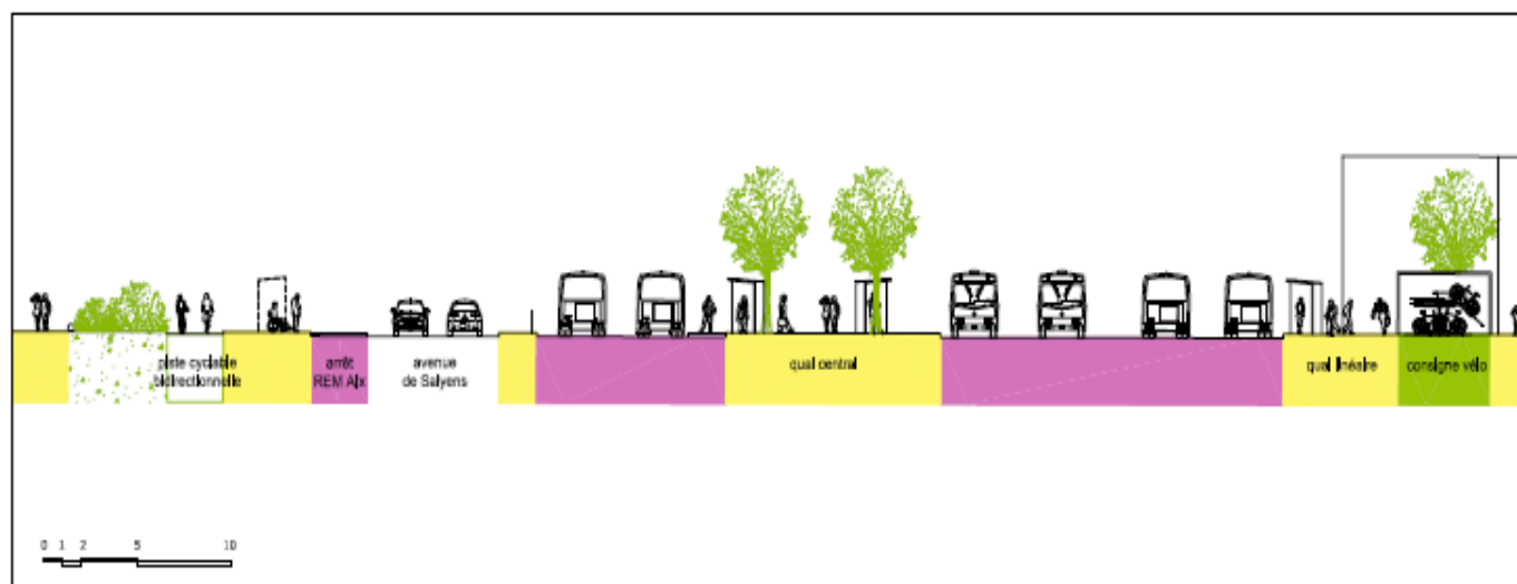
Esquisse de réorganisation - coupe transversale
